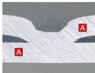
接合断面観察
