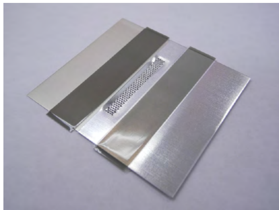
上: [アルミタブ t =0.4 mm] 下: [Niめっき銅タブ t =0.2 mm]
