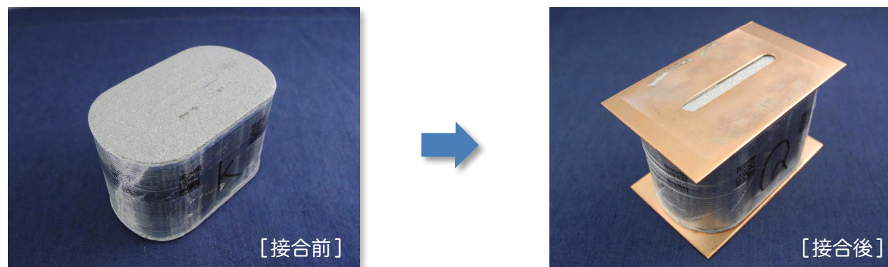
[超大型フィルムコンデンサの亜鉛層と銅電極板の両面接合]
