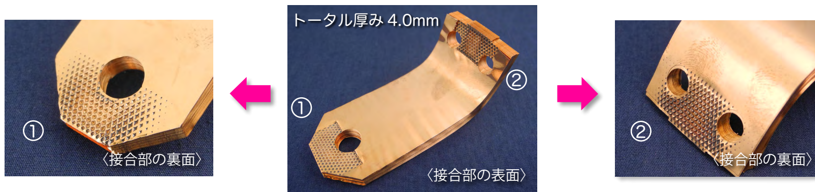
[銅シート(厚み 0.1mm) 40枚のマルチ接合]
