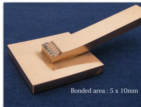
★ [厚さ 4mm] 銅バー & 銅ブロック
