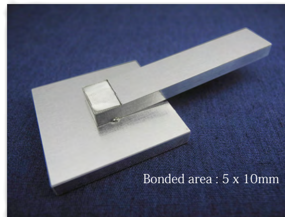
★ [厚さ 4mm] アルミバー & アルミブロック
